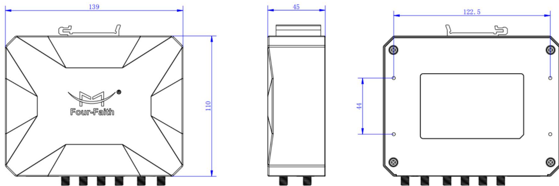
5G 工业路由器尺寸
