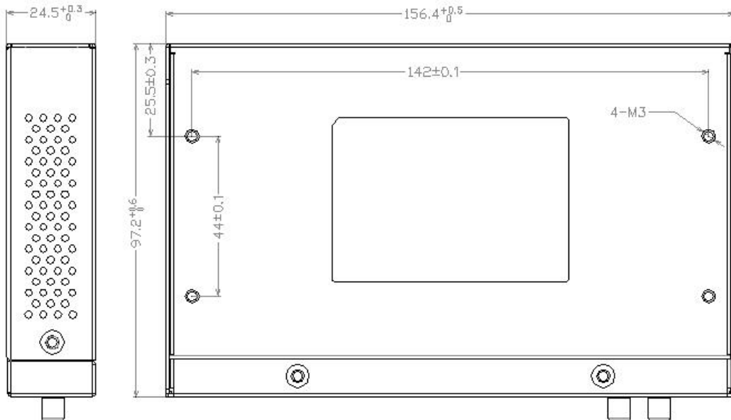
路由器尺寸
